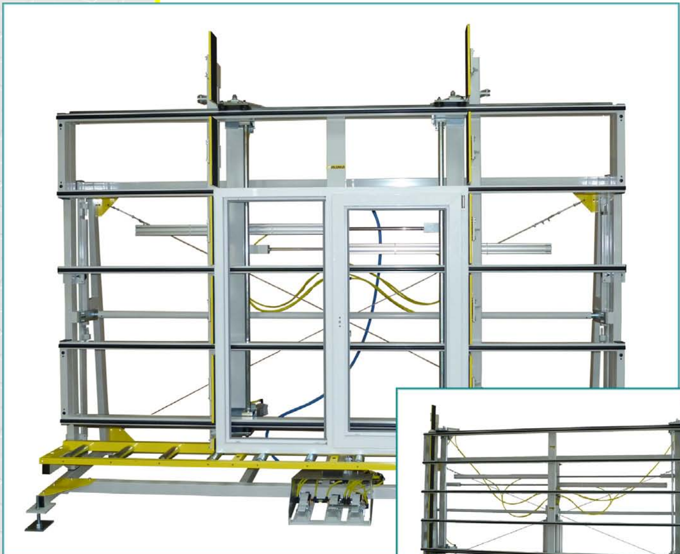
Kontrolná a zasklievacia jednotka FIXUS D
