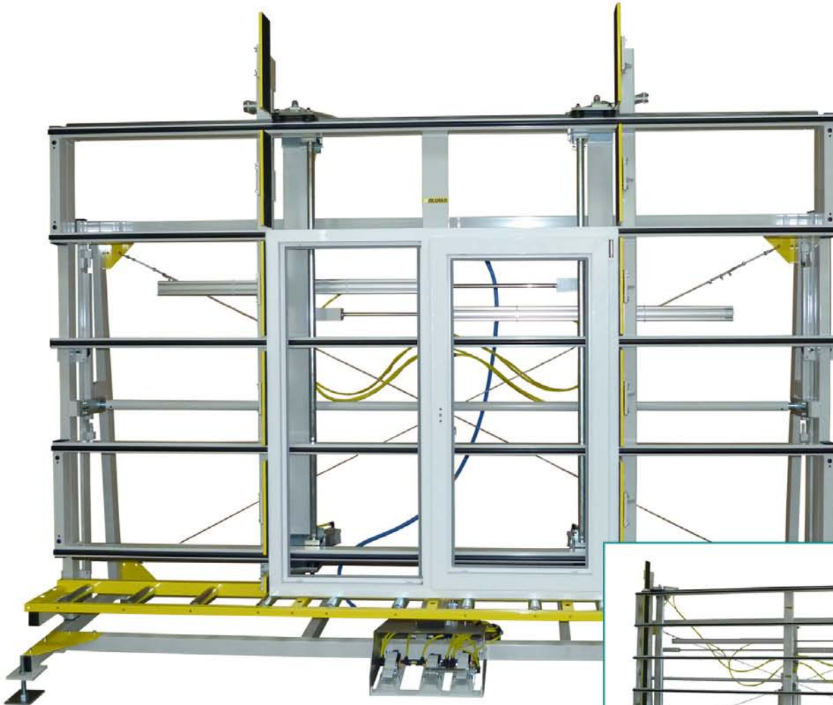
Kontrolna stanica i Platforma za stakljenje FIXUS D
