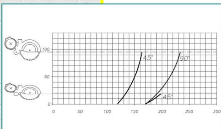
Řezný diagram NORMA 350
