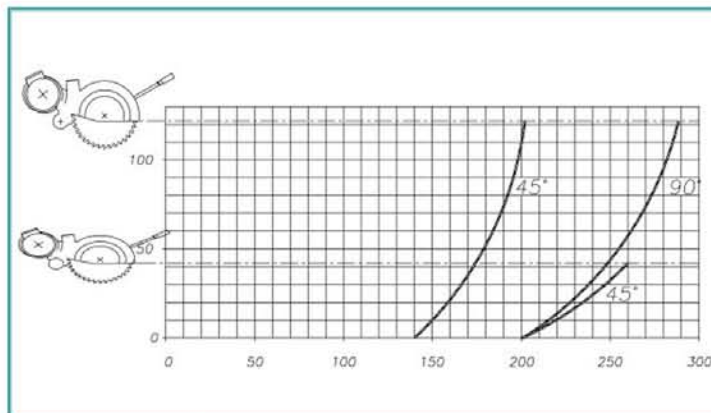
Řezný diagram NORMA 400
