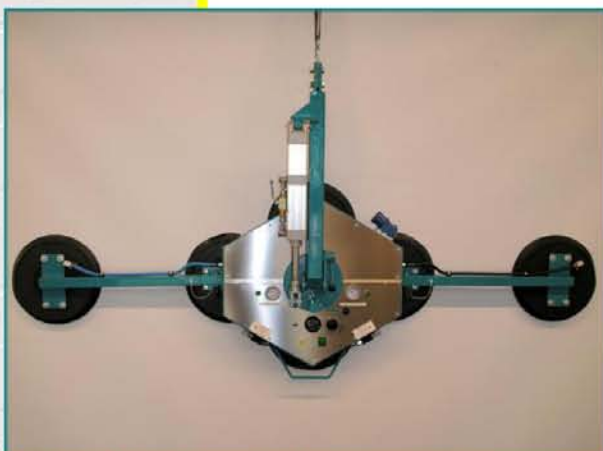
Részlet a függőleges és vízszintes helyzetben történő mozgásra
