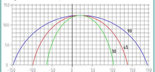
Vágástartomány LMS 350 GM / GMPV
