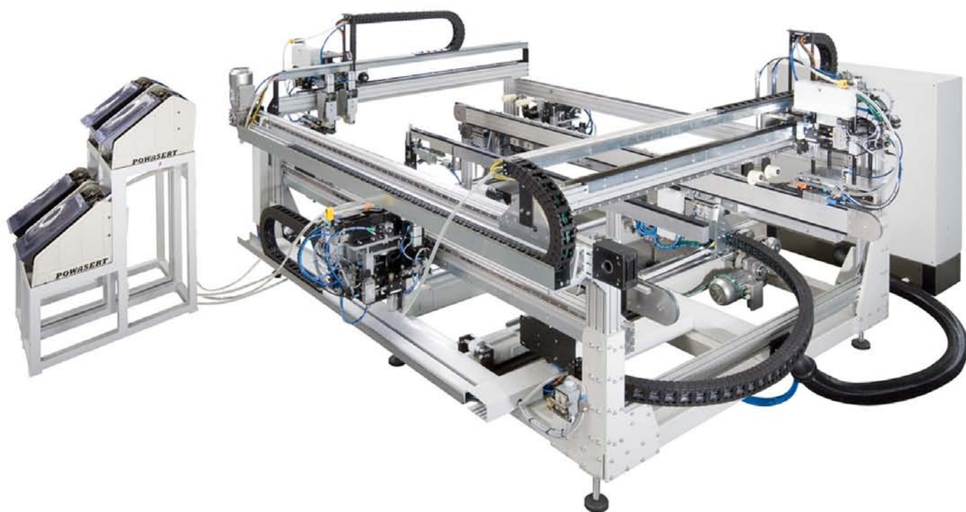
FBS-1M - Automatický skrutkovač na priskrutkovanie dielov kovania do krídla
