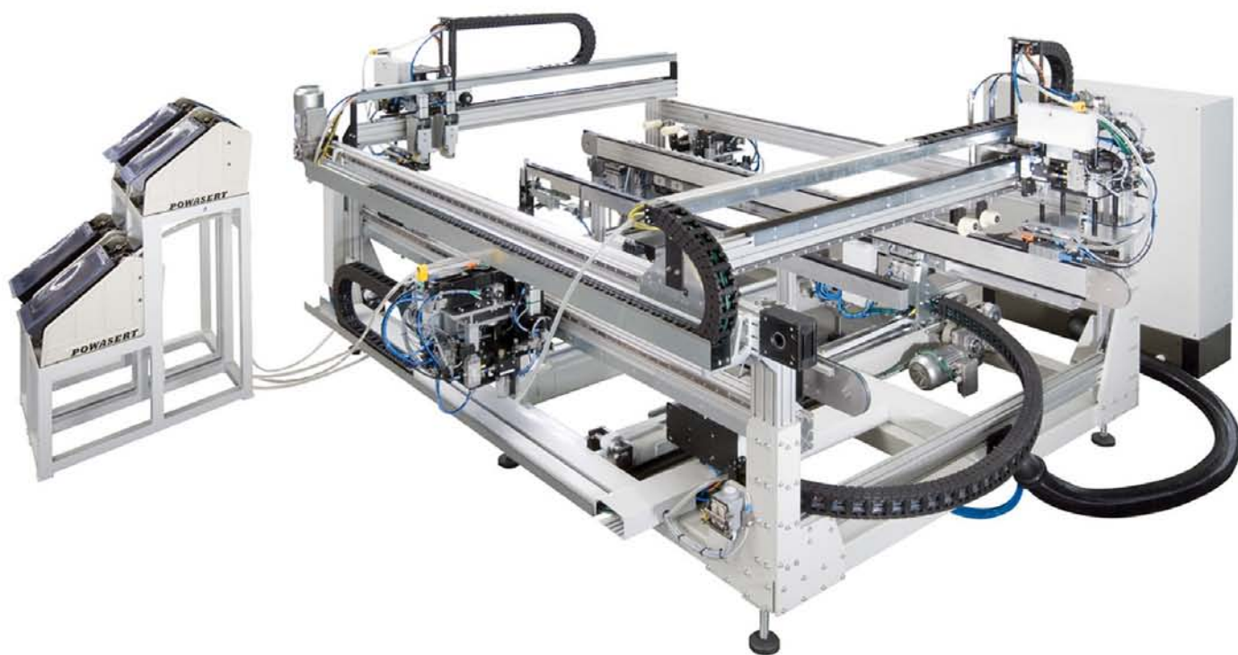
FBS-1M – Автоматический шуруповёрт для привинчивания частей фурнитуры на створку
