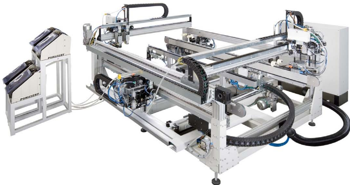
FBS-1M - Automatický šroubovák na přišroubování dílů kování do křídla
