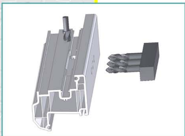
Opracovanie profilu
