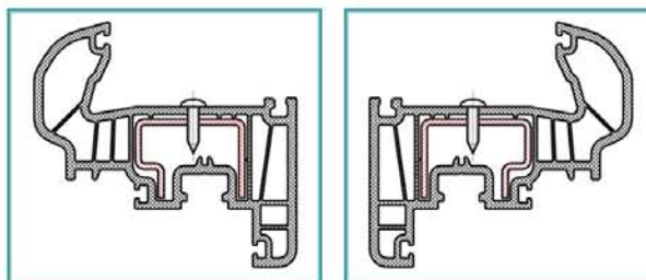
Закрепление армирующего профиля ADS DE 1/1
