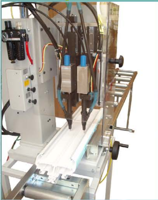
Šroubovák výstuží ADS DE 1/1
