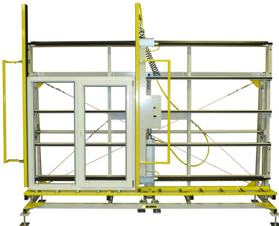
Kontrolná a zasklievacia jednotka FIXUS S (so zdvihom ľavý)
