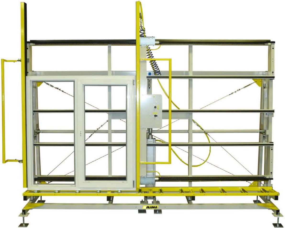
Kontrolna stanica i platforma za zastakljivanje FIXUS S
