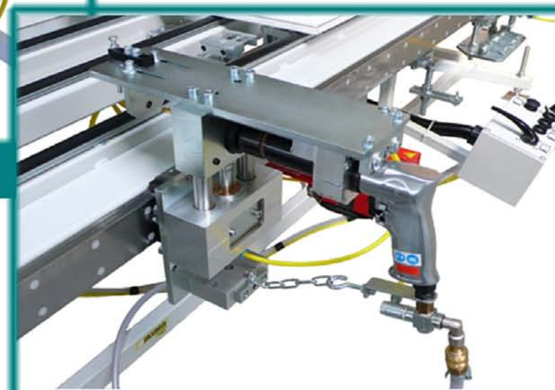
Mozgatható fűróegység
