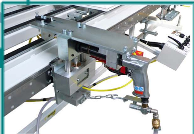
Unité de vissage déplaçable
