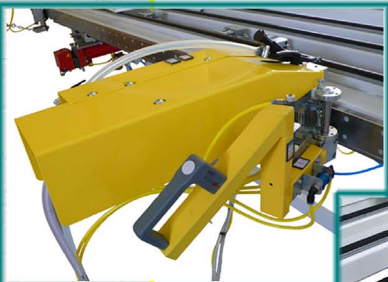
Tournevis déplaçable avec aménagement automatique des vis
