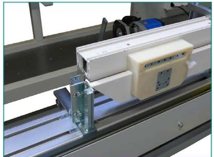
uložení rámu a křídla symetricky překládací doraz
