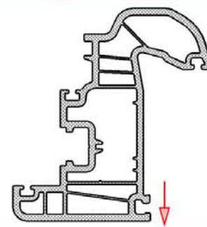
Зачистка внутреннего угла в месте установки штапика
