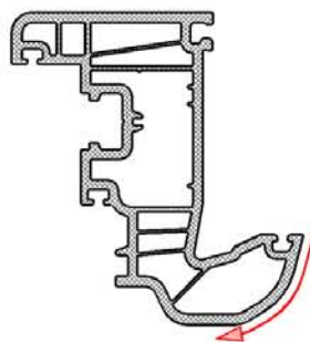
Зачистка внутренних углов для любого типа профиля
