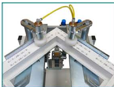
Čišćenje spoljnog luka ( radijusa) sa lakoćom COMBI RADIUS
