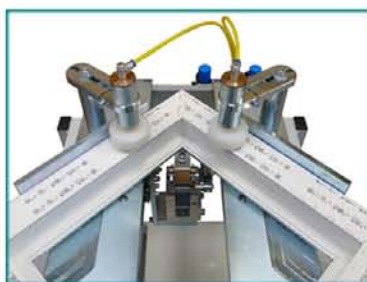
COMBI RADIUS berendezés a belső sarkak letisztításához
