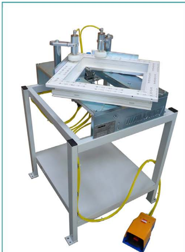
COMBI RADIUS berendezés a belső sarkak letisztításához
