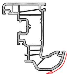
Bármilyen alakzatú profil belső sarkának letisztítása
