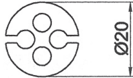
Gumový profil - žltý obj. č.: 91-8AV 020 028
